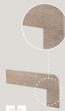
Zanquín Recto dcha./izda. 42,3 x 17,5 cm - 16.92"x 7"
