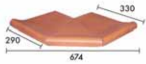
(*) CARTABÓN BORDE PISCINA EXTERIOR
