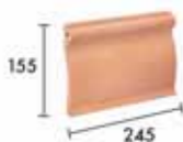
REMATE DE FRISO
