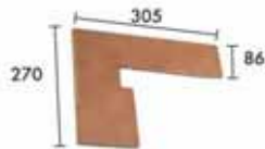
ZANQUÍN RECTO
